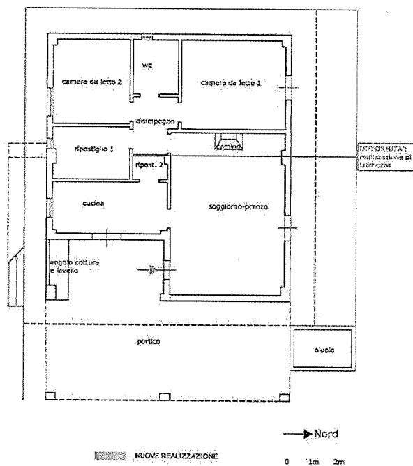
Planimetria di rilievo attuale con indicazione delle difformità rispetto al grafico di progetto autorizzato (All. 26)
