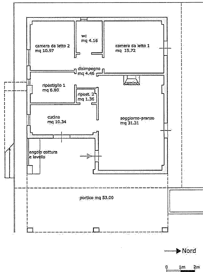
Planimetria di rilievo dello stato di fatto (All. 12)
